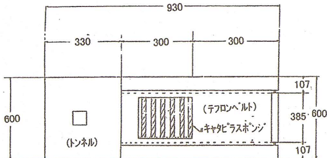
機械寸法図
